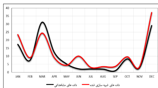
شکل (۲). شبیه‌سازی داده‌های مشاهداتی بارش برای پیش‌بینی RCP26
