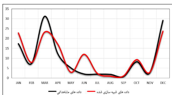
شکل (۳). شبیه‌سازی داده‌های مشاهداتی بارش برای پیش‌بینی RCP45
