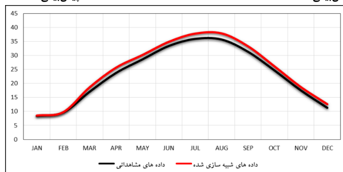
شکل (۱۰). شبیه سازی داده های مشاهداتی حداکثر دما برای پیش بینی RCP85
