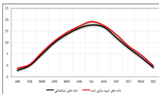
شکل (۶) شبیه سازی داده های مشاهداتی حداقل دما برای پیش بینی RCP45
