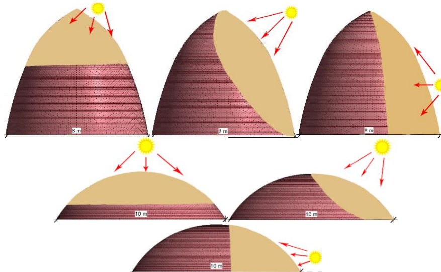
شکل (۱۰). از سمت بالا تصاویر گرافیکی میزان دریافت تابش بر سطوح گنبد خیز بلند در سه بازه‌ی زمانی روز (۱۳، ۱۴، ۱۶). از سمت پایین تصاویر گرافیکی میزان برخورد تابش خورشید بر سطوح گنبد آب‌انبارهای خیز کم در سه بازه‌ی زمانی روز (۱۳، ۱۴، ۱۶). منبع: نگارندگان.
