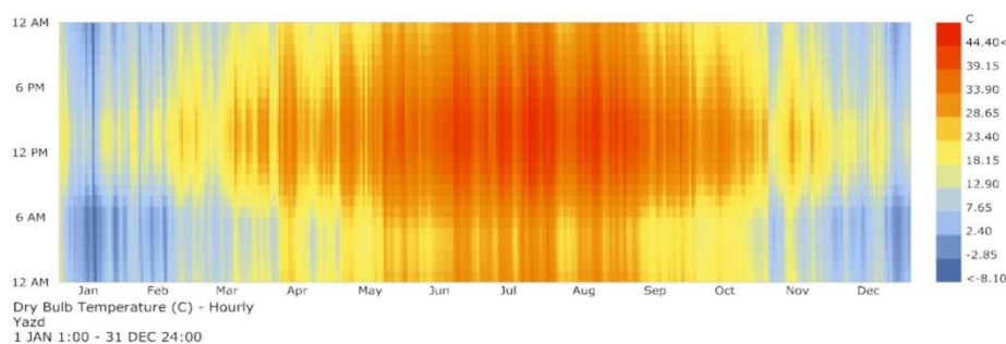
شکل (۲). دمای خشک سالانه اقلیم شهر یزد که بالاترین دما در طول سال ۴۴ درجه سانتی‌گراد و پایین‌ترین دما ۸- درجه سانتی‌گراد می‌باشد. منبع: هانی‌بی لیدی باگ، نگارندگان.
