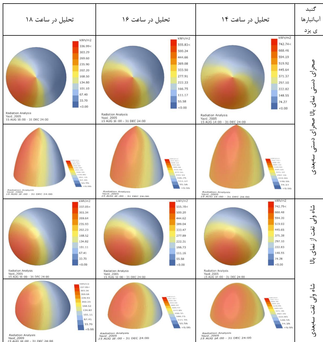
شکل (۵). تحلیل دریافت تابش خورشید، جذب حرارت در محدوده سایه بر سطوح گنبد آب‌انبارهای یزد بر حسب
