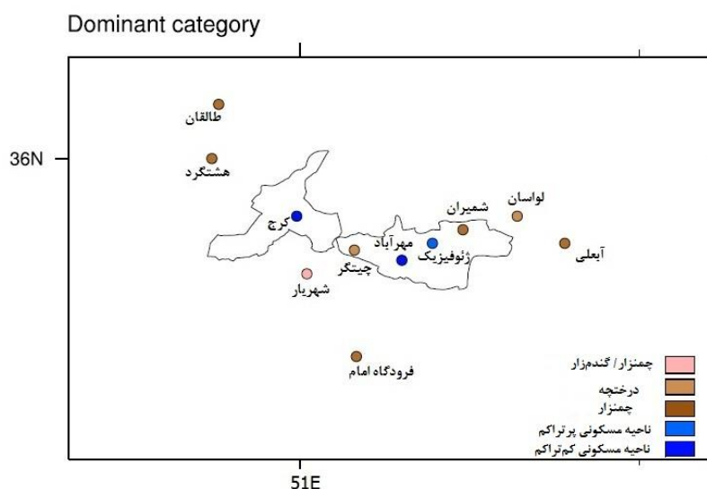
شکل (۲). کاربری اراضی ایستگاه‌های مورد مطالعه با اجرای سه کلاس در حوزه چهارم.
