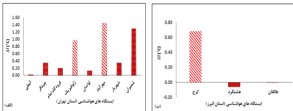
شکل (۳). اختلاف دمای هوای ۲ متری (حالت مرجع - اصلاح شده) در ایستگاه‌های هواشناسی منطقه مورد مطالعه
