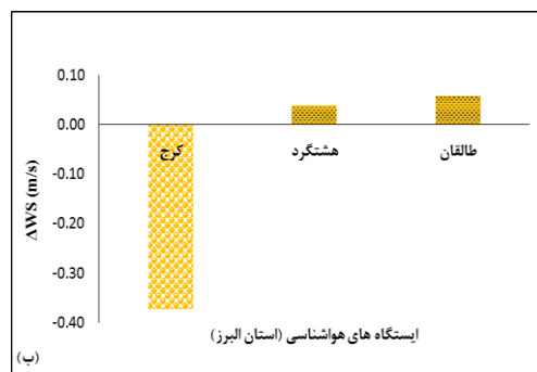
شکل (۴). اختلاف سرعت باد ۲ متری (حالت مرجع - اصلاح شده) در ایستگاه‌های هواشناسی مناطق مورد مطالعه
