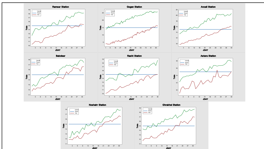
شکل (۱۰): نمودار مقایسه رسیدن دمای کمینه ایستگاه ها به دمای پایه در شرائط فعلی و دوره شبیه سازی شده مدل و شیفت رسیدن به دمای پایه به سمت بهار و زمستان در دوره شبیه سازی
