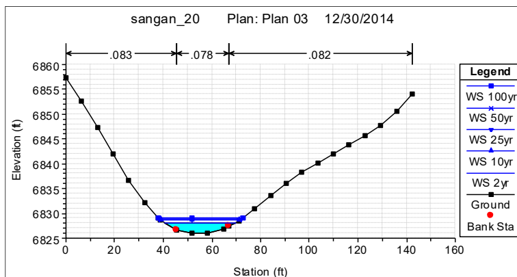
شکل (۵). ارتفاع سطح سیل گیر به ازای دوره بازگشت‌های گوناگون در ابتدای بازه
