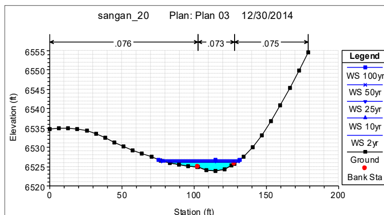
شکل (۶). ارتفاع سطح سیل گیر به ازای دوره بازگشت‌های گوناگون در بازه B
