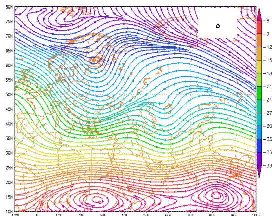
شکل (۱۲). نقشه‌های میانگین وزش دمای الگوهای الف: اول، ب: دوم، ج: سوم، د: چهارم، ه: پنجم
