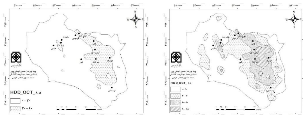
شکل (۸). پراکنش مکانی نیازهای گرمایشی مهر، دوره
