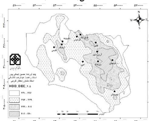
شکل (۱۶). پراکنش مکانی نیازهای گرمایشی آذر در دوره
