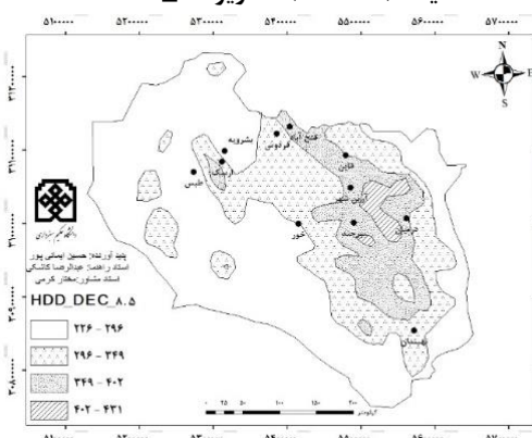
شکل (۱۵). پراکنش مکانی نیازهای گرمایشی آذر در دوره
