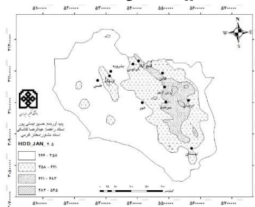
شکل (۲۰). پراکنش مکانی نیازهای گرمایشی ماه دی در دوره آینده (۲۰۱۶-۴۱)، سناریو RCP_4.5
