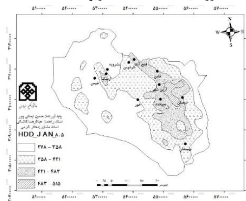
شکل (۲۱). پراکنش مکانی نیازهای گرمایشی ماه دی در دوره آینده (۲۰۱۶-۴۱)، سناریو RCP_8.5
