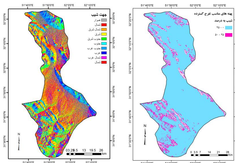
شکل (۶). نقشه مناطق مستعد تفرج
