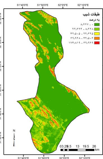
شکل (۴). نقشه شیب
