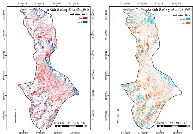
شکل (۸). مناطق مستعد طبقه یک تفرج
