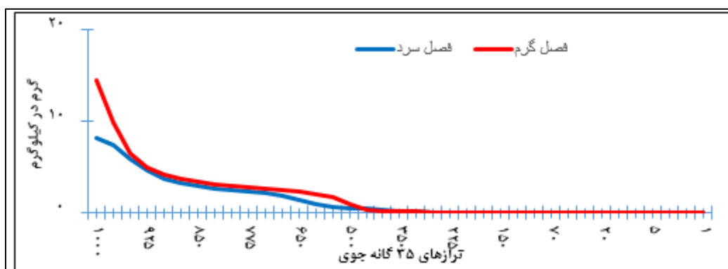
شکل (۱۲). توزیع عمودی رطوبت ویژه جو در ترازهای ۳۵ گانه جو منطقه به تفکیک فصل سرد و گرم (براساس داده های با اندازه پیکسل ۰/۱۲۵ درجه قوسی پایگاه داده ECMWF، نسخه Era-Intrim)
