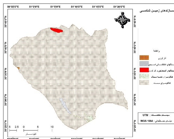
شکل (۱۰): سازندهای زمین منطقه مورد مطالعه
