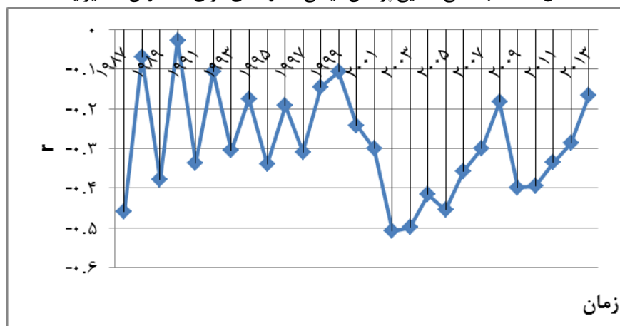
شکل (۱۰). همبستگی فضایی پوشش گیاهی (r) و دمای هوای ماه آوریل
