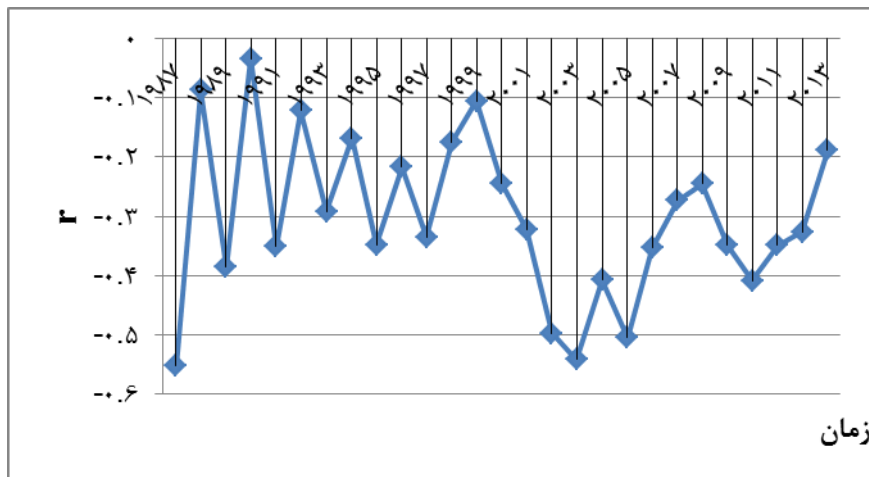
شکل (۹). همبستگی فضایی پوشش گیاهی (r) و دمای هوای ماه مارس (تأخیر یک ماهه)
