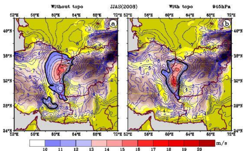
شکل (۹). شدت باد در شرایط با توپوگرافی (راست) و بدون توپوگرافی خراسان شمالی، رضوی و جنوبی (چپ) در تراز بیشینه سرعت باد (۹۴۵ ه.پ.). پربند سیاه پررنگ نشان‌دهنده سرعت باد ۱۰ متر بر ثانیه است.
