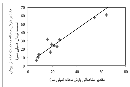
شکل (۵). مقادیر محاسباتی بارش ماهانه به‌دست آمده از روش نسبت نرمال نسبت به مقادیر مشاهده‌ای
