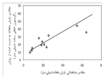
شکل (۲). مقادیر محاسباتی بارش ماهانه به‌دست آمده از روش رگرسیون خطی ساده نسبت به مقادیر مشاهده‌ای
