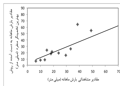
شکل (۶). مقادیر محاسباتی بارش ماهانه به‌دست آمده از روش بهترین تخمین گر منفرد نسبت به مقادیر مشاهده‌ای
