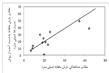
شکل (۷). مقادیر محاسباتی بارش ماهانه به‌دست آمده از روش نسبت‌ها نسبت به مقادیر مشاهده‌ای
