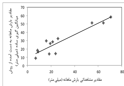
شکل (۴). مقادیر محاسباتی بارش ماهانه به‌دست آمده از روش میانگین‌گیری ساده نسبت به مقادیر مشاهده‌ای
