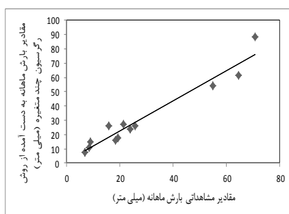
شکل (۳). مقادیر محاسباتی بارش ماهانه به‌دست آمده از روش رگرسیون چند متغیره نسبت به مقادیر مشاهده‌ای
