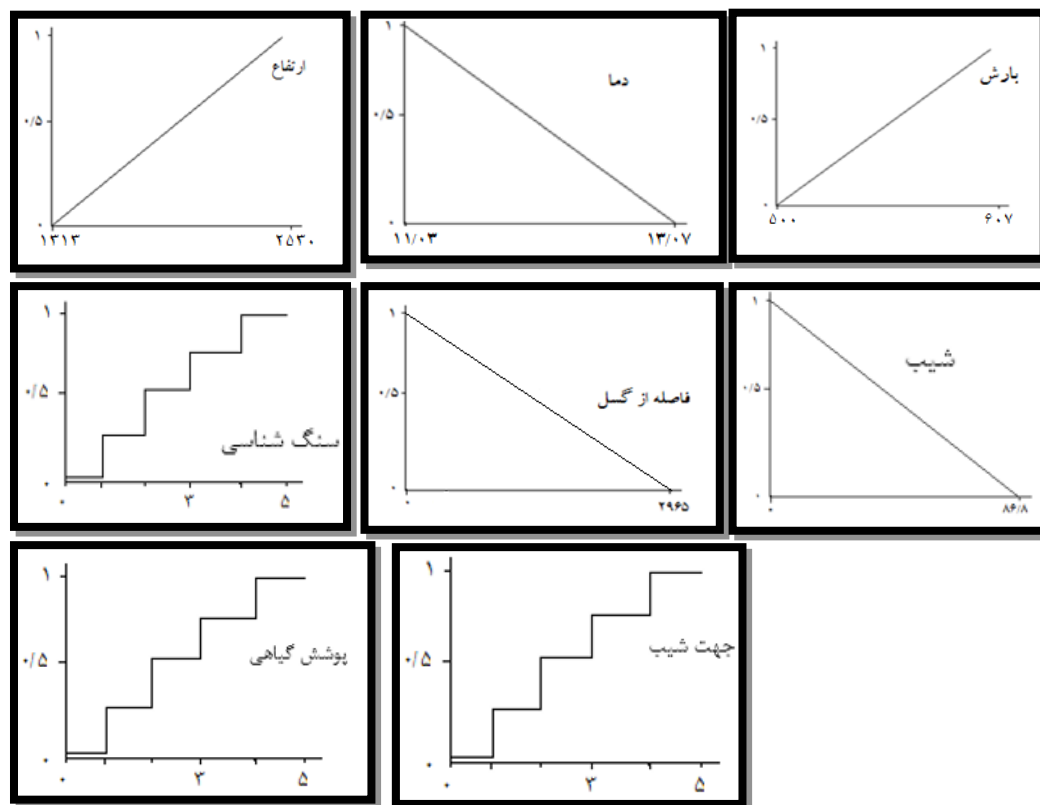
شکل (۲) نمودارهای تابع فازای هر یک از عوامل موثر در توسعه کارست منطقه مورد مطالعه
