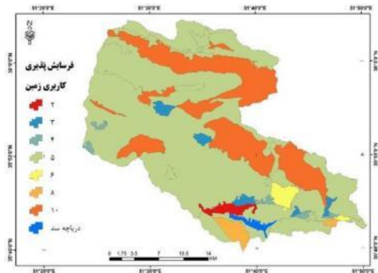
شکل (۳). نقشه حساسیت انواع کاربری از نظر فرسایش
