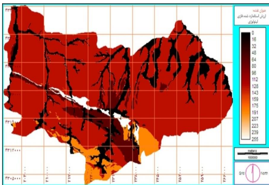
شکل (۵). نقشه استاندارد شده تغییرات زمین‌شناسی سازندها (فشاری تک محوری)
