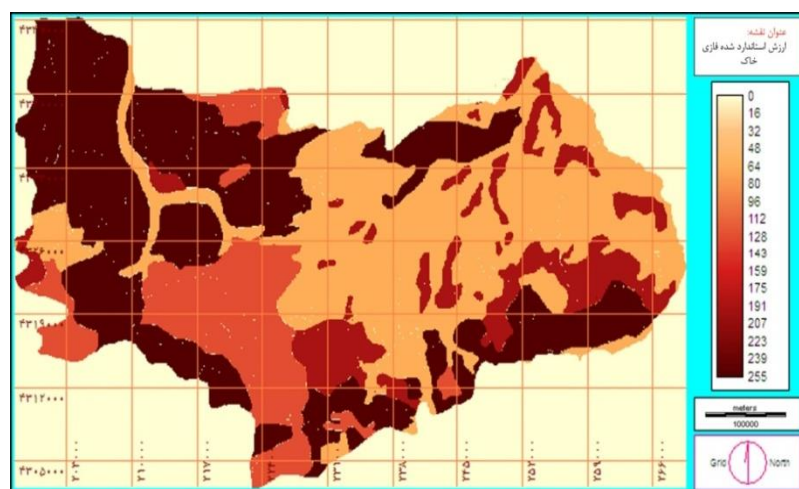
شکل (۱۱). نقشه استاندارد شده خاک
