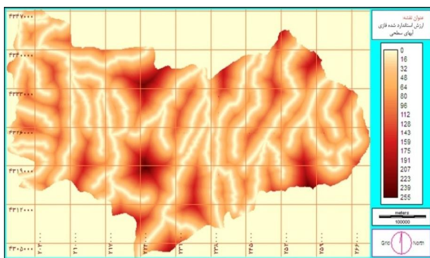
شکل (۴). نقشه استاندارد شده‌ی فاصله از آبراه
