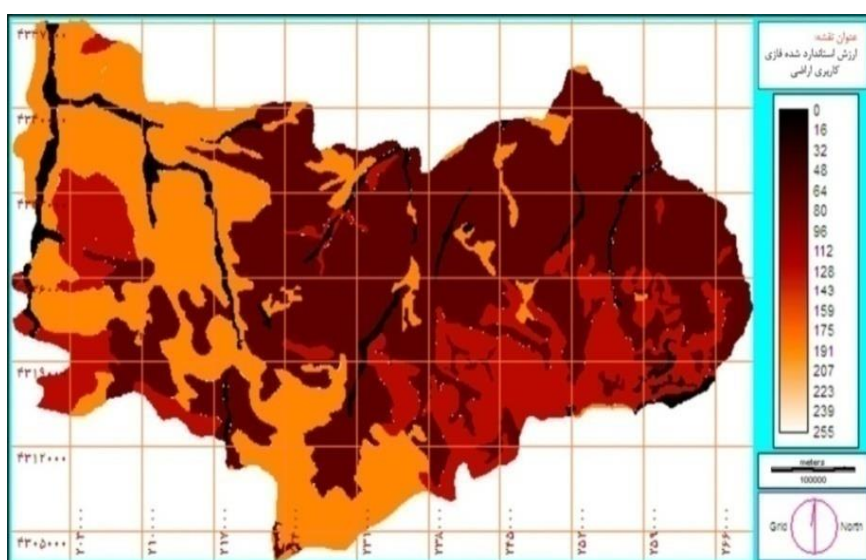
شکل (۸). نقشه استاندارد شده فازی بارش (میل‌متر)
