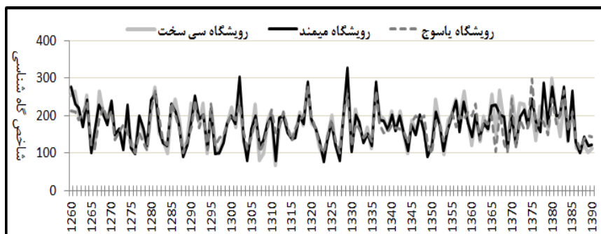
شکل (۳) نمایش میانگین شاخص گاه شناسی رویشگاه های سی سخت، میمند و یاسوج در جنگل های بلوط ایرانی منطقه دنا در رشته کوه های زاگرس مرکزی ایران، طی ۱۳۱ سال گذشته (۱۳۹۰-۱۲۶۰)
