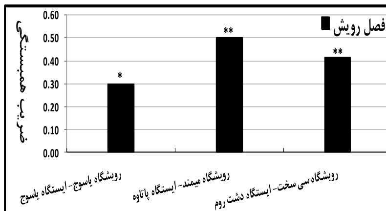
شکل (۵) رابطه میان میانگین دمای اردیبهشت - شهریور، با گاه شناسی رویشگاه های منطقه دنا
