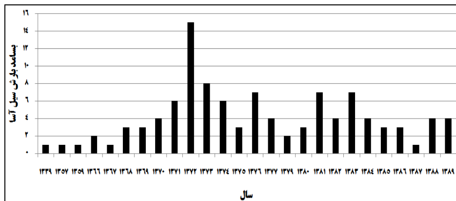
شکل (۲) بسماند سالانه‌ی رخداد بارش‌های سیل‌آسای استان کردستان برپایه‌ی آستانه‌ی صدکی ۹۸ (برحسب درصد) و فراگیری
