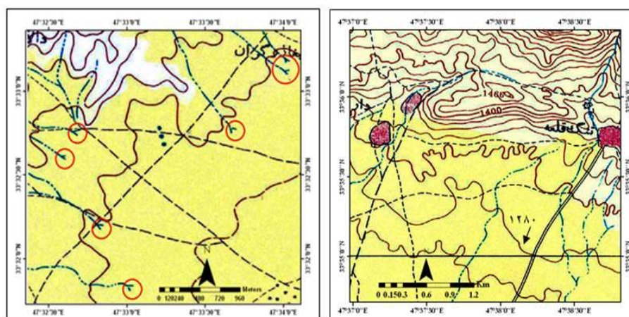
شکل (۱۴) تغییر فرم خطوط منحنی میزان (۱۵) توزیع آبراهه‌های دوشاخه در دشت کوهدشت
