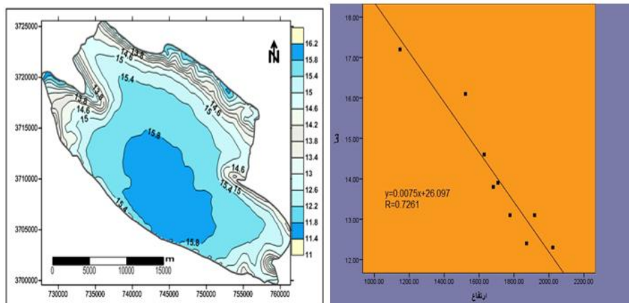
شکل (۶) رابطه دما با ارتفاع در زمان حاضر
