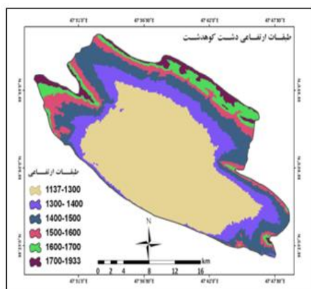
شکل (۱۱) تصویر Google earth ارتفاعات کوهدشت شکل (۱۲) طبقات ارتفاعی حوضه مورد مطالعه
