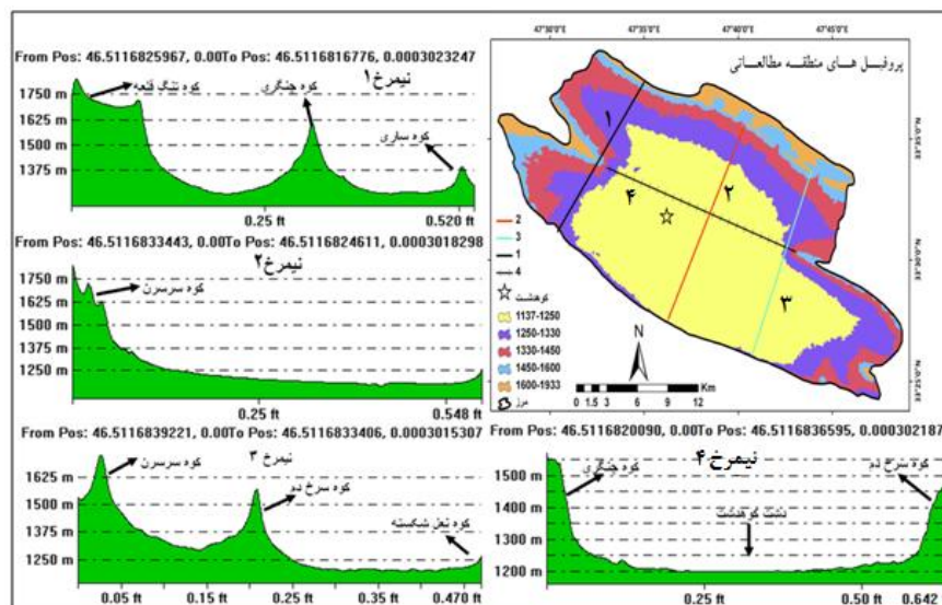
شکل (۳) نیمرخ‌های چهارگانه دشت کوه‌دشت
