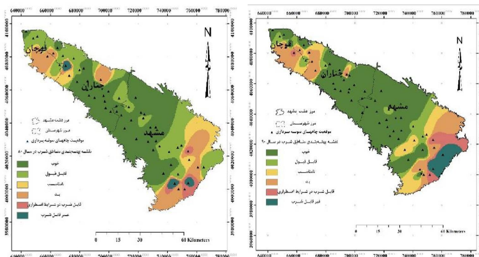
شکل (۷) پهنه بندی کیفیت آب شرب دشت مشهد در سال ۱۳۸۰ (راست) و ۱۳۹۰ (چپ)
