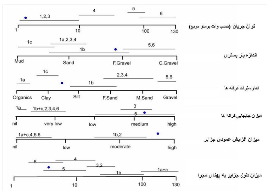
شکل (۱۱) طبقه‌بندی شماتیکی نانسون و نایتون (۱۹۹۶) برای رودخانه‌های آدا و موقعیت رودخانه مهاباد در این طرح، توجه کنید چگونه رودخانه مهاباد نتوانسته با این طرح مطابقت نماید.
