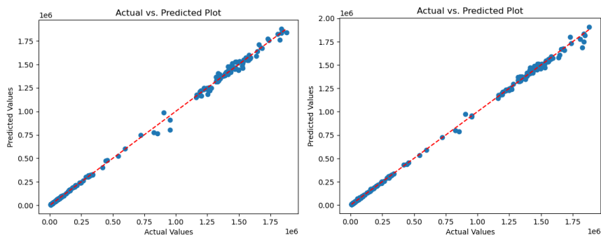
شکل ۵. نمودار پراکندگی RF
