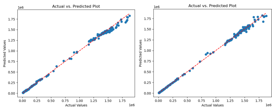
شکل ۷. نمودار پراکندگی HGB
