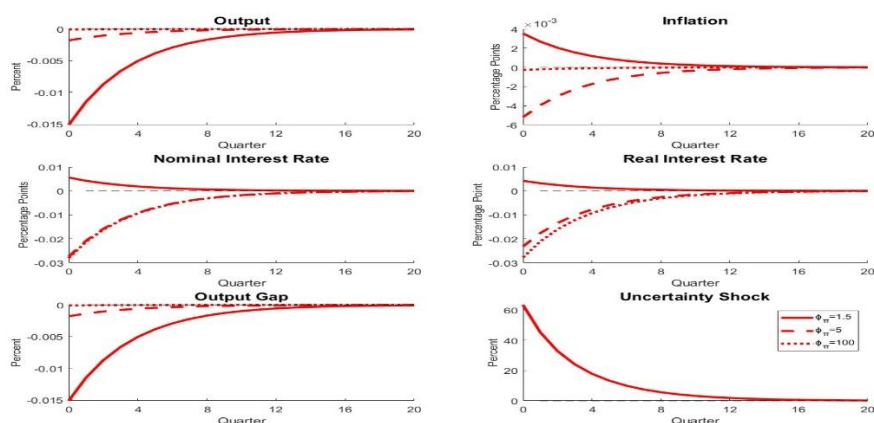
شکل ۳-۴. نمودار توابع عکس العمل ضربه‌ای به تکانه‌های عدم قطعیت تحت قواعد تیلور (کالوو) منبع: یافته‌های تحقیق
