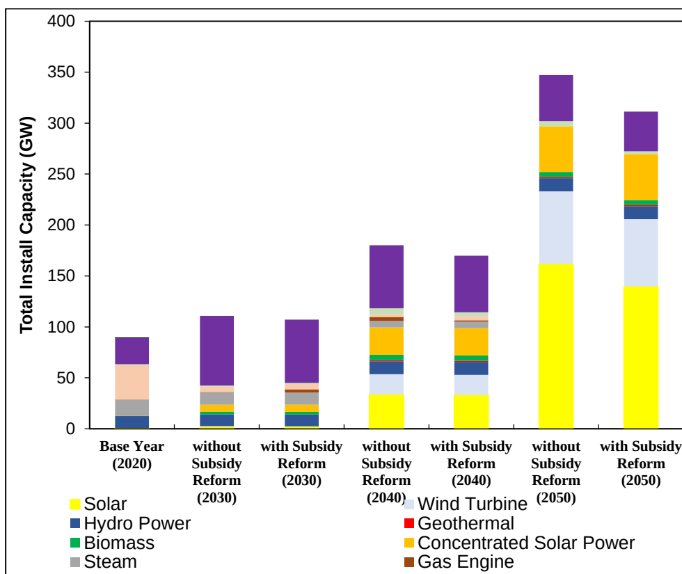
نمودار ۸. کل ظرفیت نصب‌شده طی سناریوهای مختلف در افق مطالعه
