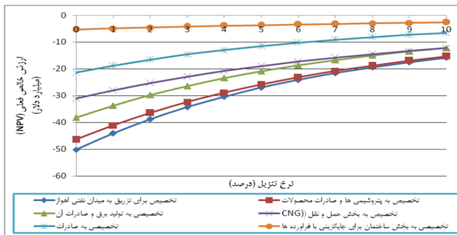
نمودار (۲) تغییرات شاخص خالص ارزش فعلی ۱ (NPV) سناریوهای مختلف تخصیص گاز طبیعی با تغییرات نرخ بهره
