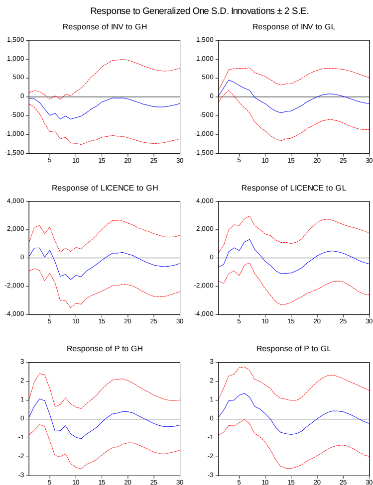
شکل ۱- توابع واکنش ضربه ای حاصل از مدل FAVAR
