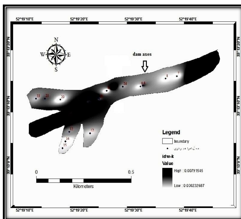
شکل ۹. نقشه نفوذپذیری آبرفت‌های سطح مخزن
