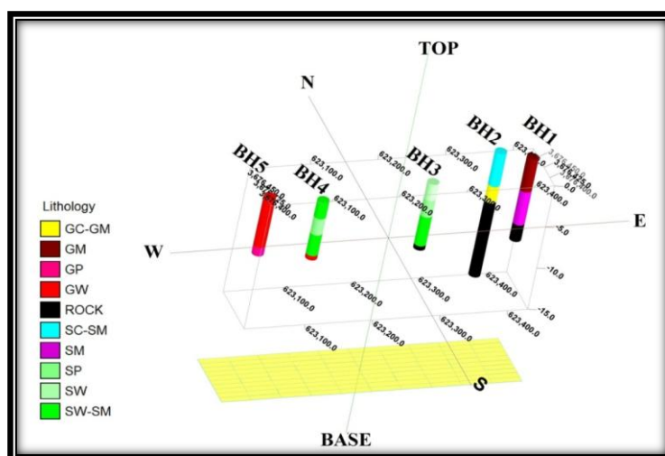
شکل ۳. موقعیت گمانه‌ها و نوع خاک تشکیل دهنده آن‌ها
