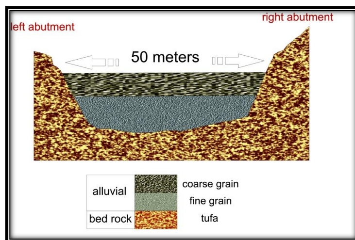
شکل ۶. نمایی از رسوبات در محل محور با توجه به نتایج به‌دست آمده از ژئوالکتریک
