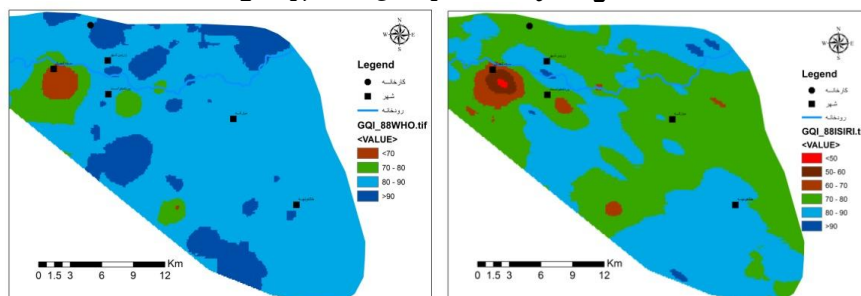
شکل ۴. پتانسیل شاخص کیفیت آب استاندارد سازمان بهداشت جهانی (WHO) (الف) و استاندارد تحقیقات صنعتی ایران (ISIRI)، (ب) منطقه پژوهش
