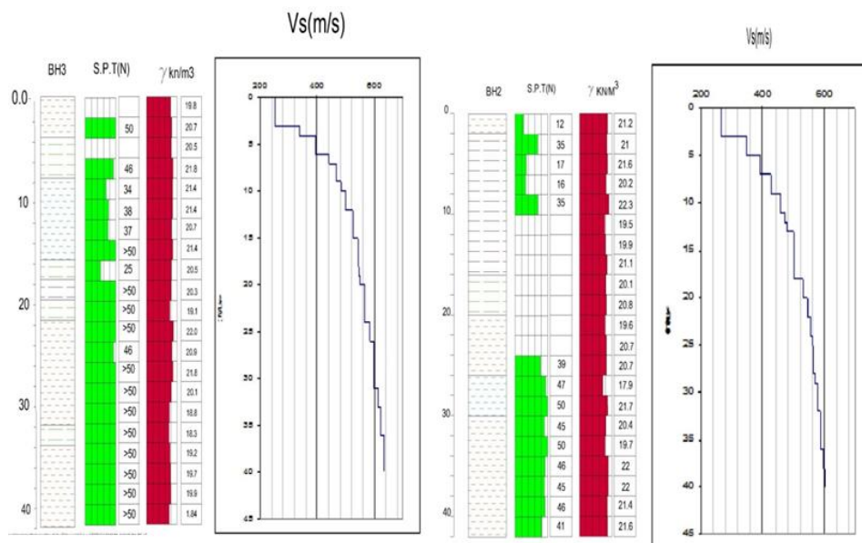
شکل ۳. پروفیل ژئوتکنیکی و ژئوفیزیکی گمانه ۲
