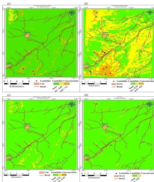
شکل ۱۳. تراکم خطر زمین‌لغزش‌های ناشی از زلزله محاسبه شده برای زلزله ۱۳۷۵ سرعین، اردبیل با M_w = 6.1 : (a) تراکم‌های پیش‌بینی شده ریزش‌ها و لغزش‌های خاکی گسسته با استفاده از کمل، (b) تراکم‌های پیش‌بینی شده لغزش‌های بلوکی و چرخشی خاکی با استفاده از کمل، (c) تراکم‌های پیش‌بینی شده لغزش‌های بلوکی و چرخشی سنگی با استفاده از کمل، (d) تراکم‌های پیش‌بینی شده جریان‌های خاکی سریع با استفاده از کمل. دایره‌های توپر زمین‌لغزش‌های رخ داده ناشی از زلزله ۱۳۷۵ سرعین، اردبیل هستند.
