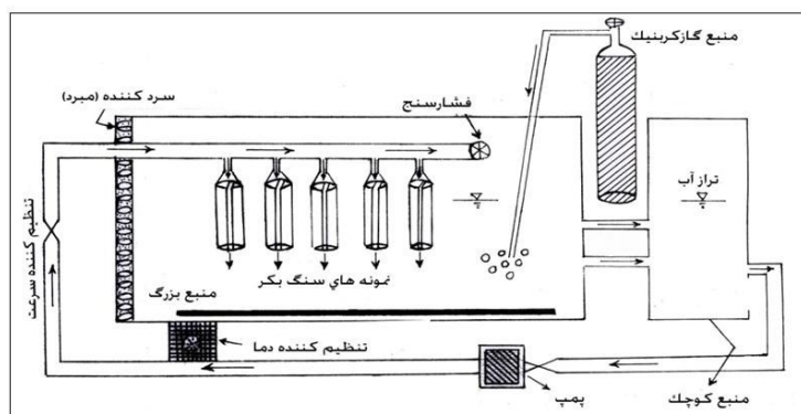
شکل ۱. طرح کلی دستگاه تعیین انحلال پذیری سنگ‌ها [۶]
