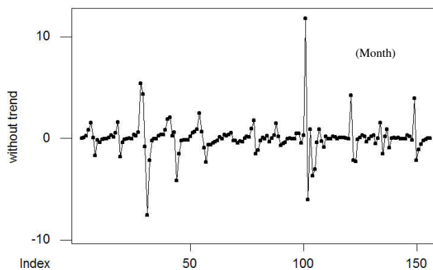
شکل ۳. حذف روند از داده‌ها از طریق معادله تفاضلی درجه یک
