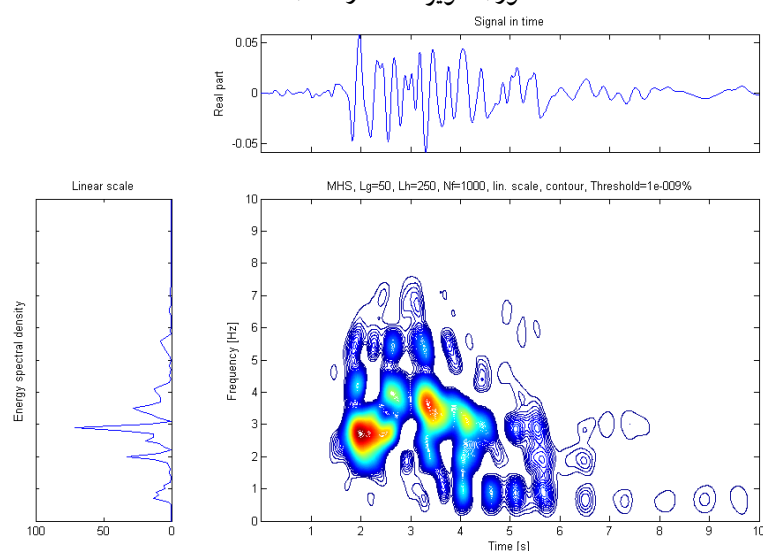
شکل ۱۱. تاریخچه زمانی شتاب‌نگاشت زلزله محاسبه شده در تاج در حالت پی با ۷۵ درصد جرم (تصویر بالا)، چگالی طیفی انرژی (تصویر سمت چپ) و تبدیل حوزه زمان - فرکانس نگاشت مذکور (تصویر سمت راست)
