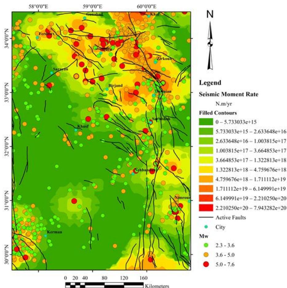
شکل ۹. نقشه پهنه‌بندی نرخ گشتاور لرزه‌ای در شرق ایران (روش IDW interpolation, power = 2) Fig. 9. Seismic moment rate zonation map of eastern Iran (IDW interpolation, power = 2)
