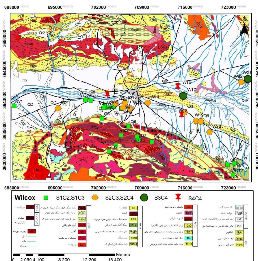
شکل ۱۱. نمودار ویلکوکس منابع آب منطقه مورد مطالعه و پراکندگی نوع منابع آب بر اساس آن
