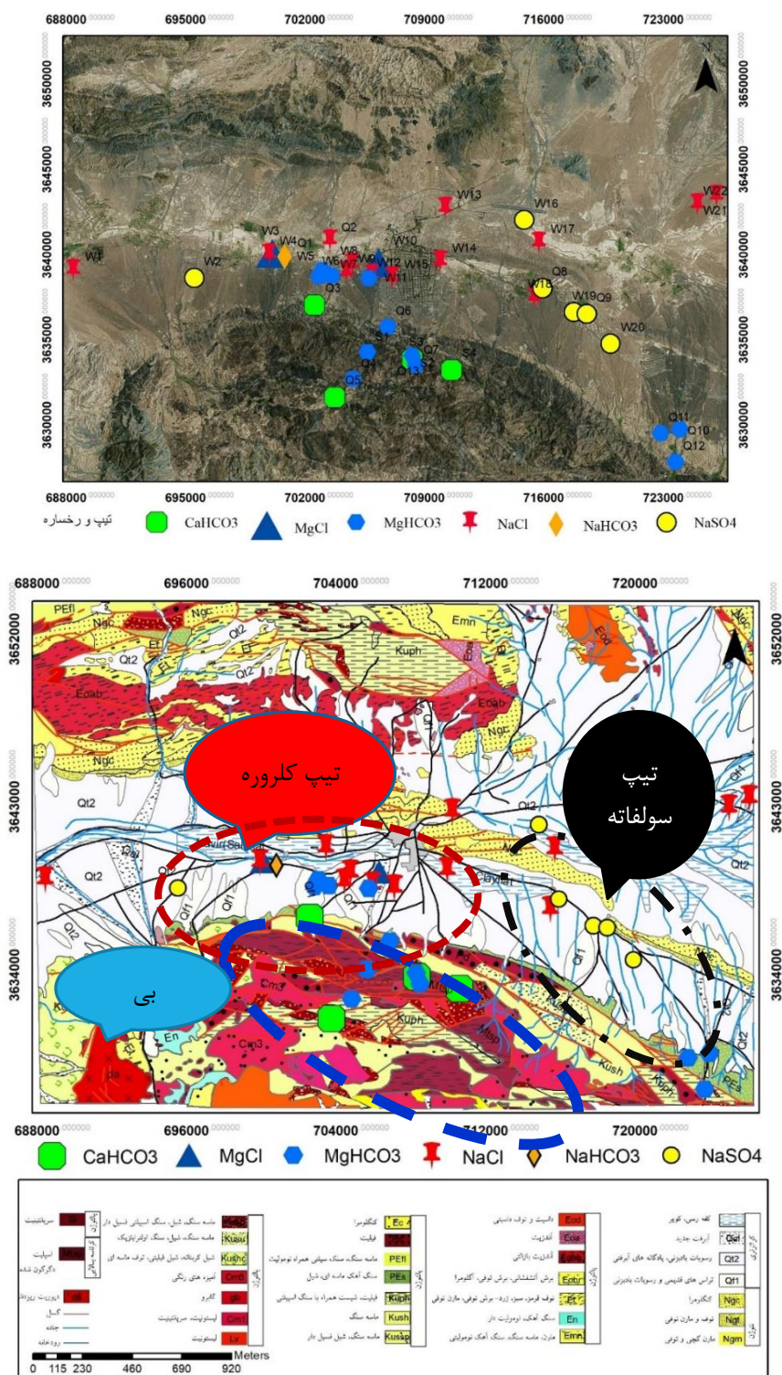
شکل ۷. نقشه توزیع پراکندگی تیپ و رخسار منابع آب منطقه مورد مطالعه Fig. 7. Distribution map of the type of water resources in the study area
