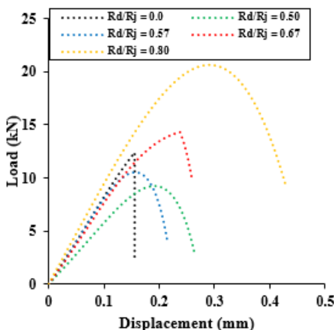
شکل ۵. تأثیر تغییر نسبت انحناء صفحات بارگذاری بر نتایج نمودار نیرو - جابه‌جایی
