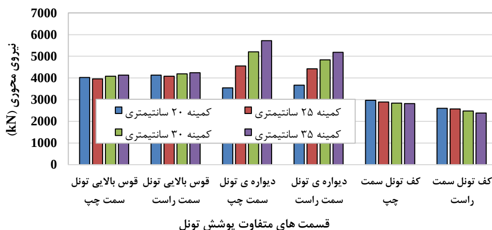
شکل ۱۳. کمینه مقادیر نیروی محوری در قسمت‌های متفاوت تونل با ضخامت متفاوت پوشش
