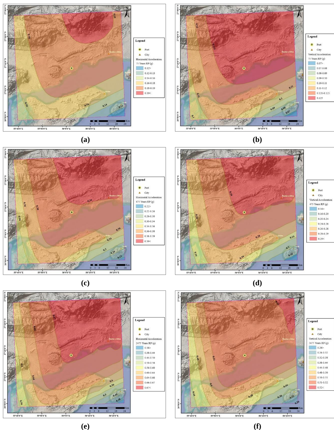
شکل ۱۰. منحنی‌های هم‌شتاب میانگین برای دوره بازگشت: (a) ۷۵ سال افقی، (b) ۷۵ سال قائم، (c) ۴۷۵ سال افقی، (d) ۴۷۵ سال قائم، (e) ۲۴۷۵ سال افقی، (f) ۲۴۷۵ سال قائم
