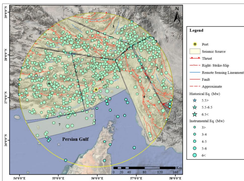
شکل ۸. چشمه‌های لرزه‌ای تعیین شده در شعاع ۲۰۰ کیلومتری بندر شهید رجایی
