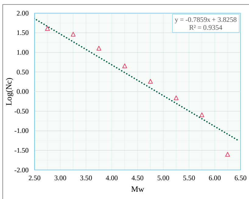
شکل ۶. رابطه خطی بین نرخ لرزه‌خیزی و بزرگا بر اساس روش گوتنبرگ - ریشتر
