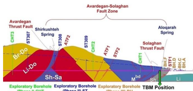
شکل ۳. مسیر تونل سبزکوه: (a) پلان، (b) پروفیل زمین‌شناسی مسیر تونل (c) محدوده مورد مطالعه (Taromi et al., 2018)
