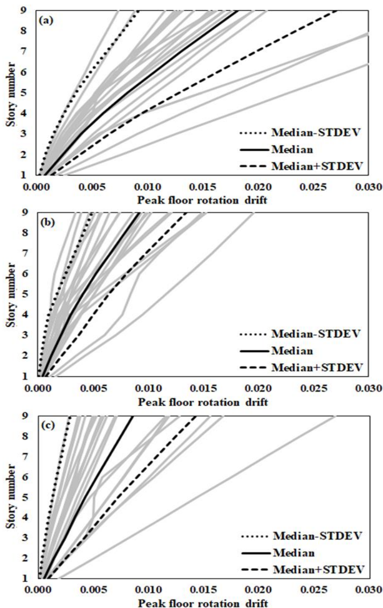
شکل ۱۳. نمودار حداکثر دریفت چرخش سقف‌های ساختمان نه طبقه در طبقات مختلف و در سطح شتاب طیفی فروریزش با e_d/A=12\% : (a) مدل آئین‌نامه‌ای، (b) مدل بالانس-۲۵٪ و (c) مدل متقارن مقاومتی
