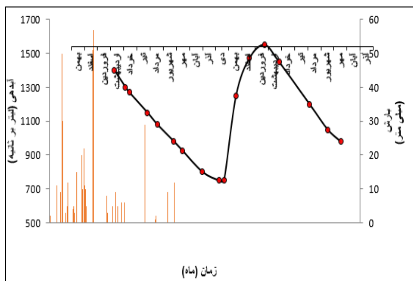
شکل ۵. هیدروگراف چشمه کارستی ورسخوران برای سال آبی ۱۴۰۲-۱۴۰۱ Fig. 5. Varsakhoran karst spring Hydrograph (the year 2022-2023)
