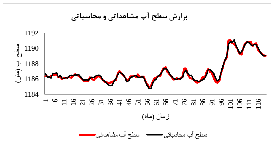
شکل ۱۳. برازش سطح آب مشاهداتی و محاسباتی طی دوره واسنجی
