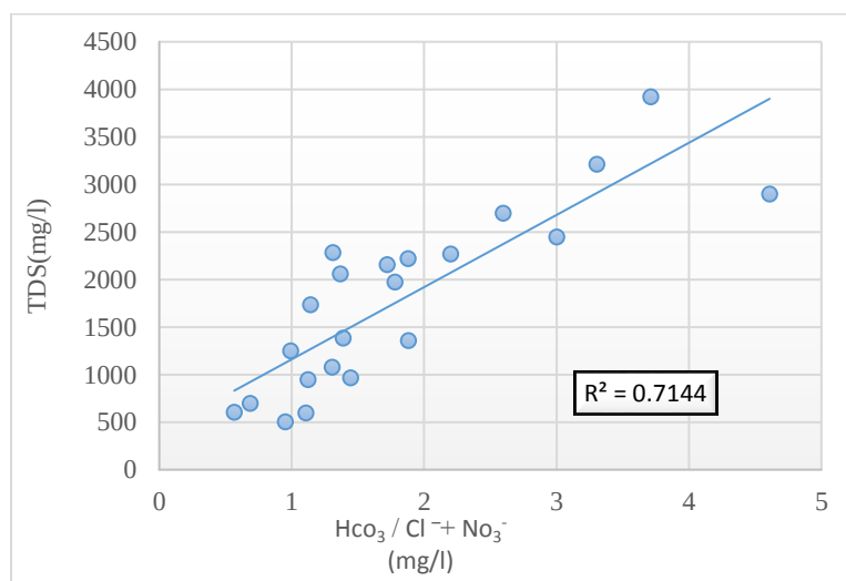
شکل ۷. نمودار نسبت یونی ( \text{HCO}_3^-/\text{Cl}^- + \text{NO}_3^- ) در مقابل (TDS)
