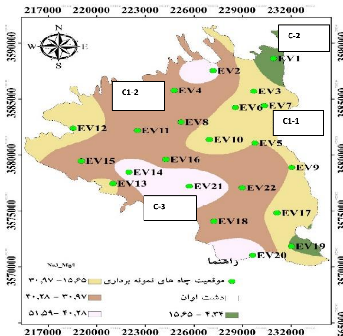
شکل ۱۰. موقعیت خوشه‌بندی سلسله مراتبی بر روی نقشه پهنه‌بندی نیترات دشت اوان
