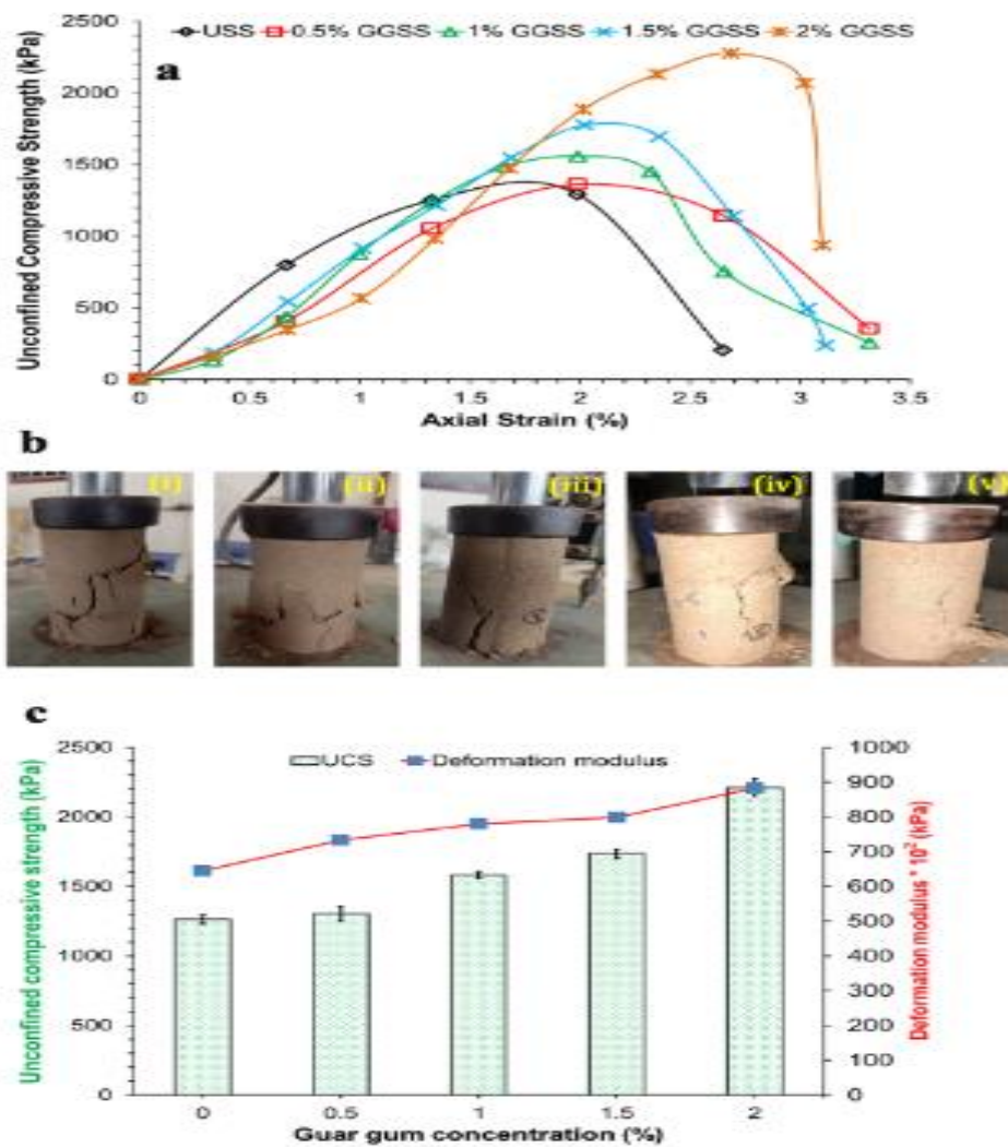
شکل ۴. مقاومت فشاری محدود نشده و رفتار خاک با غلظت‌های متفاوت بایوپلیمر زیستی گوار گام (Soldo et al., 2020).
