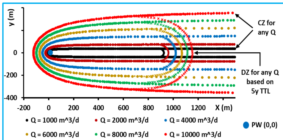
شکل ۱۲. حریم آگیر و حریم تخلیه برای مقادیر مختلف دبی پمپاژ. خطوط زمان گذر ۵ ساله هستند.
