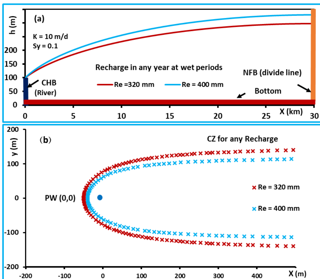
شکل ۱۵. اثر نسبت تخلیه به تغذیه بر حریم آبرگیر در چاه مرکزی آبخوان. شکل تغییر حریم آبرگیر چاهی در مرکز یک آبخوان را نشان می‌دهد که سطح تراز آن از طریق چاه‌هایی که به طور مناسب در کل آبخوان جانمایی شده‌اند تنزل یافته است. مقدار تخلیه‌ی کل چاه‌ها معادل ۸۰ میلی‌متر از کل تغذیه‌ی آبخوان بوده است.
