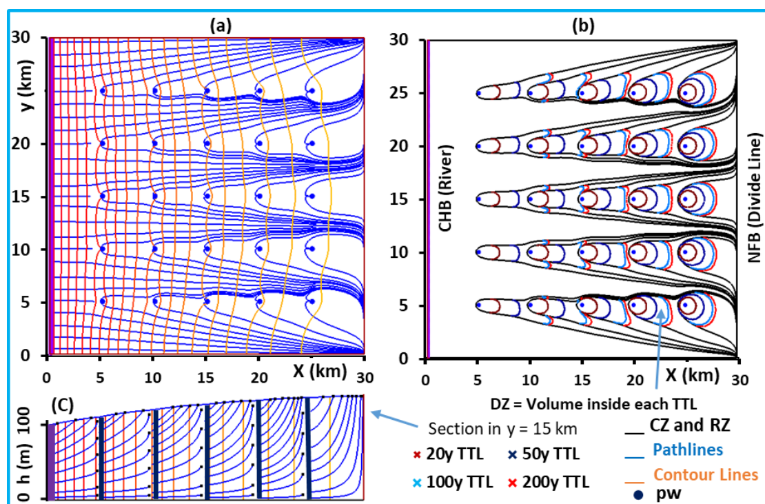
شکل ۱۴. حریم آگیر و حریم تخلیه و حریم تغذیه در یک آبخوان آزاد آبرفتی با سطح آب اولیه شیب‌دار در یک سیستم چندچاهی (حریم تأثیر هر چاه بخش عمده‌ای از کل آبخوان است)
