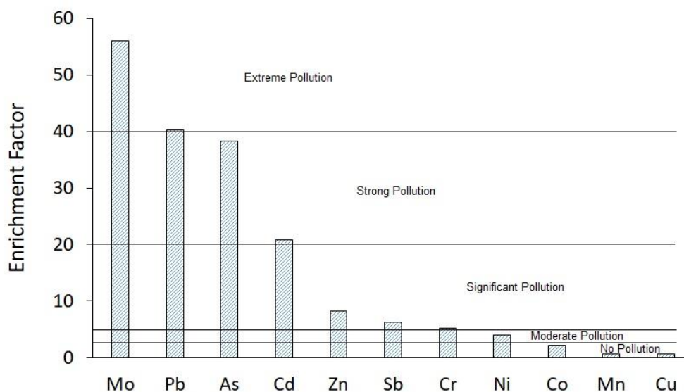
شکل ۲. رده‌بندی عناصر بالقوه سمّی در نمونه‌های باطله زغال‌شویی بر اساس مقادیر متوسط ضریب غنی‌شدگی Fig. 2. The classification of the potentially toxic elements on the coal wahery waste samples bases on the average enrichment factor values
