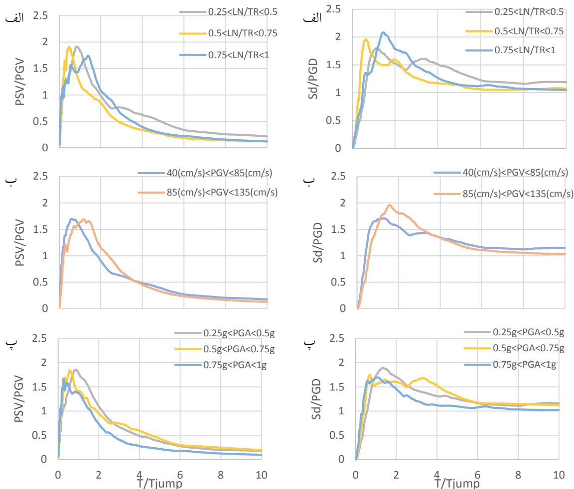
شکل ۷- طیف پاسخ جابجایی نرمال دوسویه با معیار گام T_{jump} (با نماد (BNDS(T_{jump})) پرش زمانی T_{jump} ، (با نماد (BNPVS(T_{jump})) شکل ۸- طیف پاسخ شبه سرعت نرمال دوسویه با معیار گام T_{jump} (با نماد (BNPVS(T_{jump})) پرش زمانی T_{jump} ، (با نماد (BNPVS(T_{jump}))
