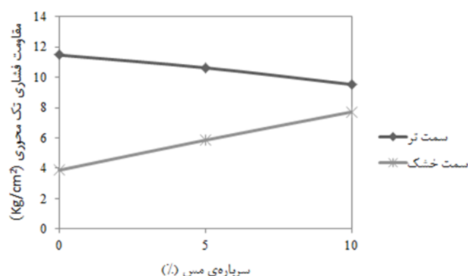
شکل ۱۸- تاثیر میزان رطوبت بر مقاومت فشاری تک‌محوری نمونه‌های با پنج درصد سیمان و کوبیده‌شده با تراکم ۹۵
