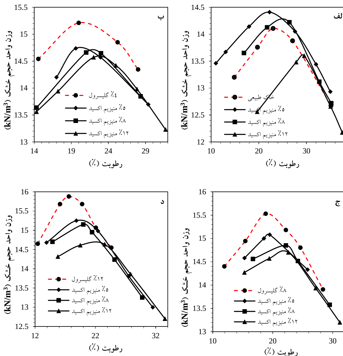
شکل ۴- منحنی تراکم استاندارد خاک طبیعی اختلاط یافته با درصد‌های متفاوت \text{MgO} و خاک آلوده حاوی درصد‌های مختلف \text{MgO}
